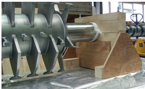
Auflager für Welle bereit zum Einschweißen.
